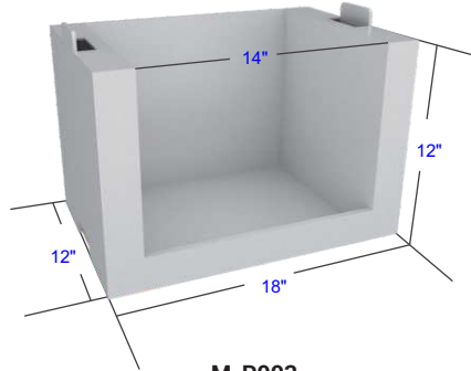
M-P003 Single PDQ
